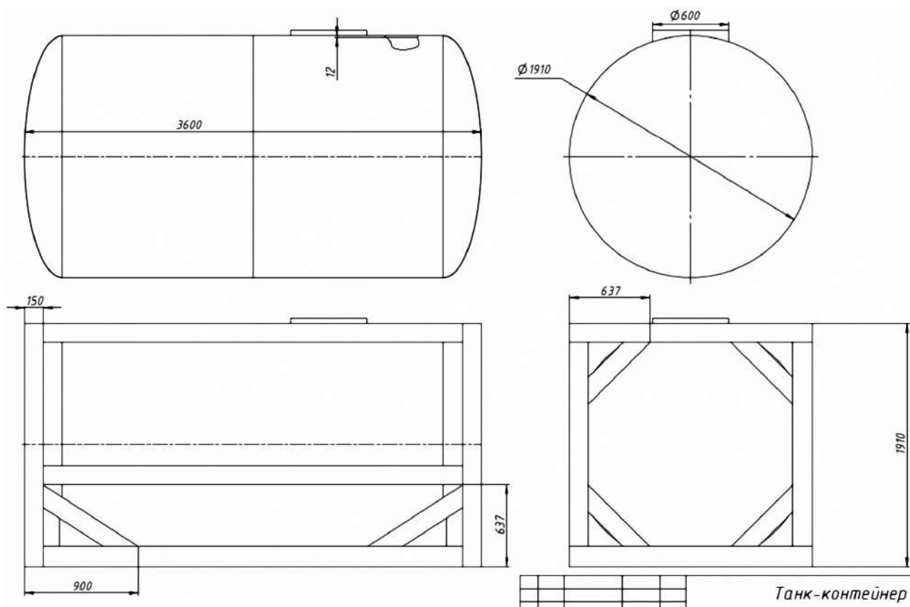
Рис. 1. Чертеж танка-контейнера в составе с полурамой
